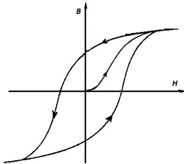
Slika 3.4. Krivulja histereze [9]
