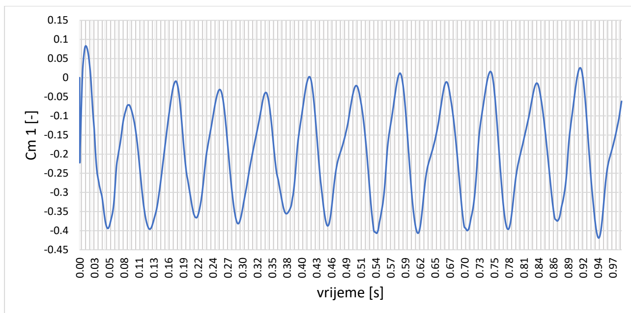
Slika 6.5. Koeficijent momenta ( C_m ) za geometriju lopatica 1
