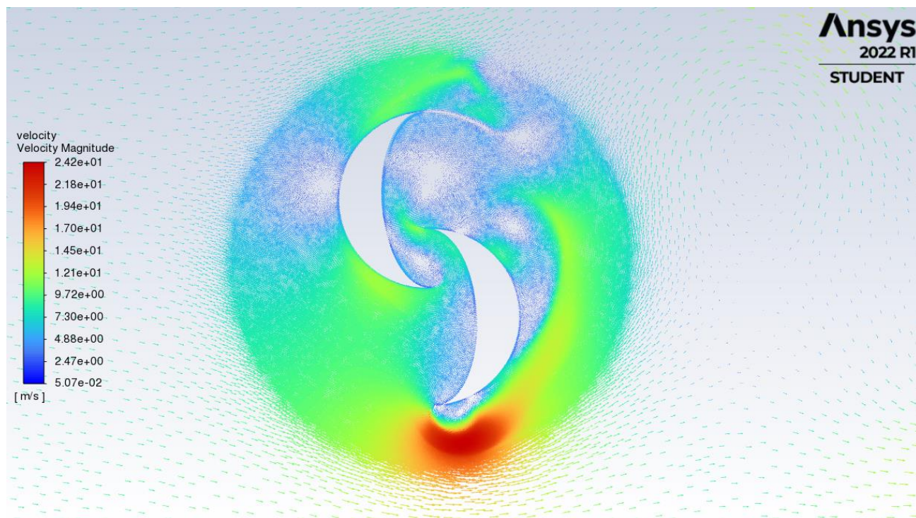
Slika 6.4. Vektori brzine geometrije lopatica 1
