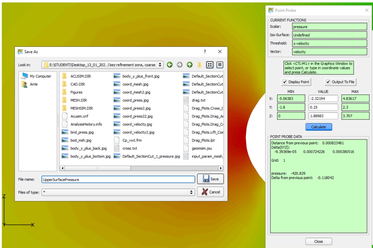
Slika 3.24 Naredba „Probe“
