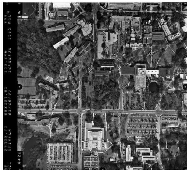
Slika 3.2 Prikaz orbitalne fotogrametrije lijevo [9], te aerofotogrametrije desno [10] (ortofoto)
