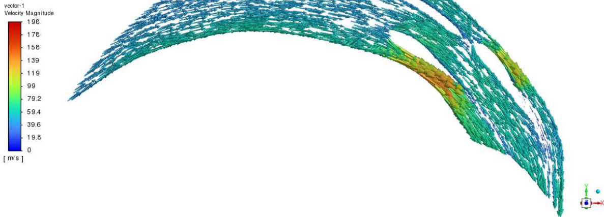
Slika 7.5 Vektori brzina za maksimalno otvoreni položaj privodećih lopatica
