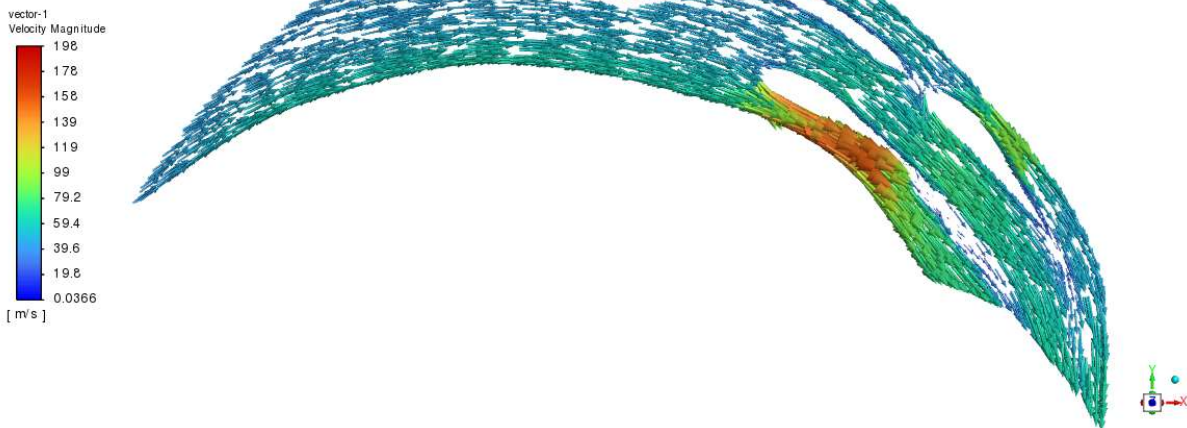
Slika 7.6 Vektori brzina za 5° od maksimalnog položaja privodećih lopatica
