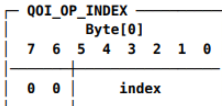
Slika 2.3 Blok bitova koji se zapisuju u 2. slučaju, preuzeto iz [9]
