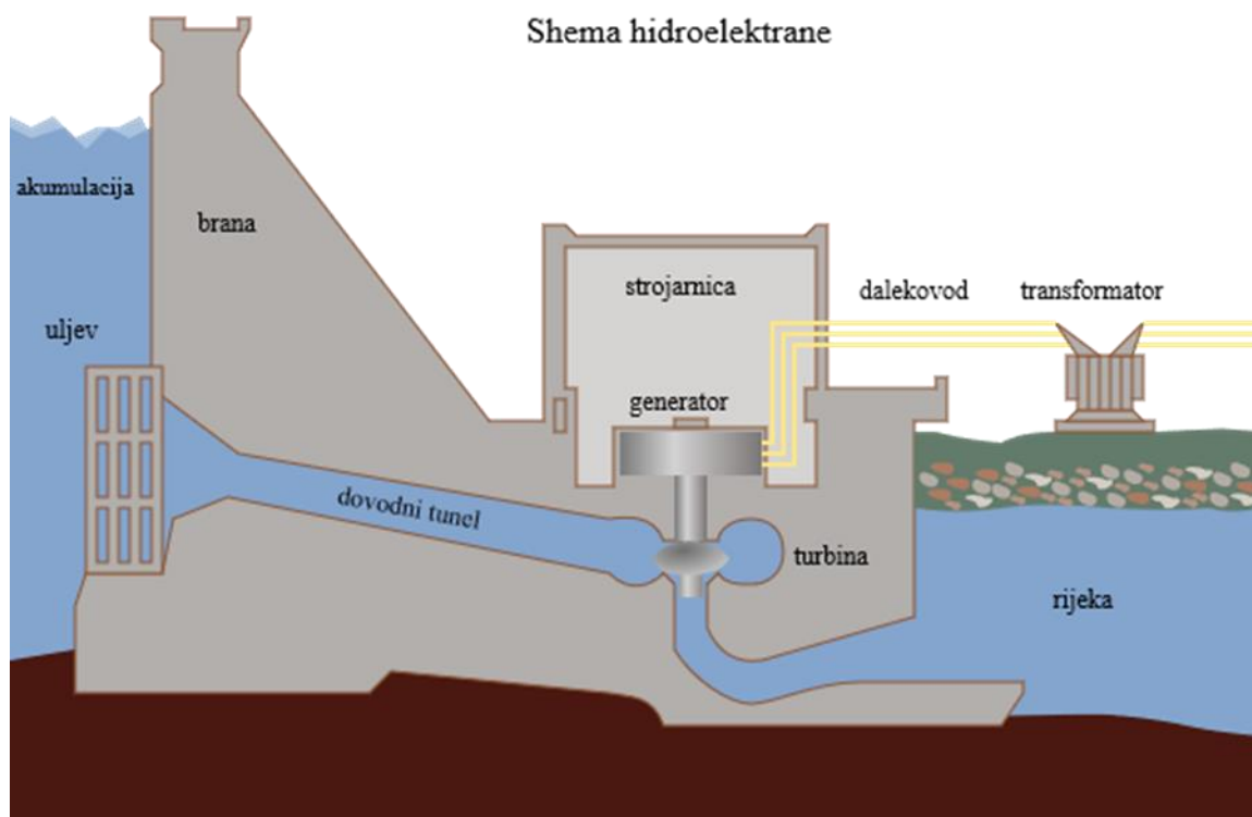
Slika 3.1. Shema hidroelektrane [13]
