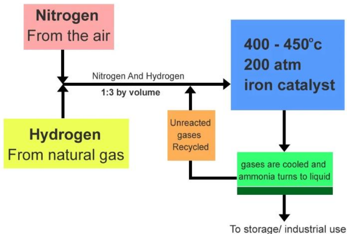
Slika 2.1. Haber-Bosch postupak [1]
