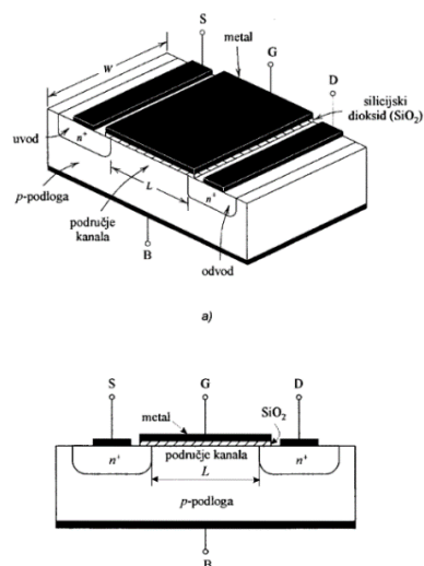
Slika 2.9 Izgled n-kanalnog MOSFETA
