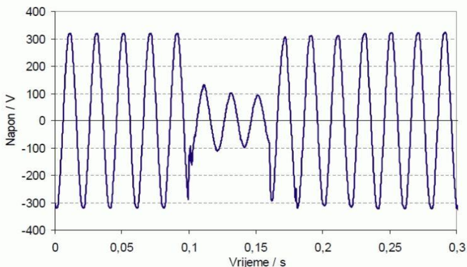
Slika 2.3. Propad napona
