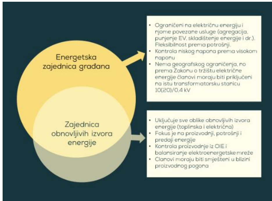
Slika 7. Energetske zajednice građana i zajednice obnovljivih izvora energije [9]
