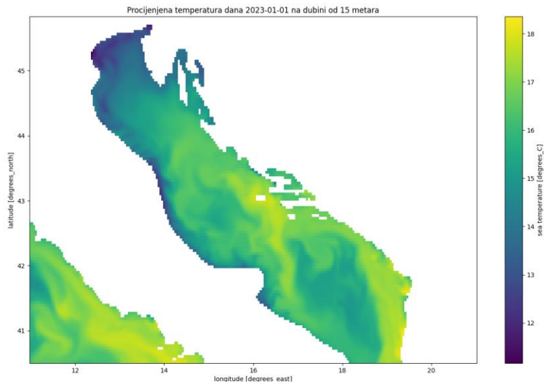
Slika 5.3.1. Termalna karta Jadranskog mora na dan 1.1.2023.
