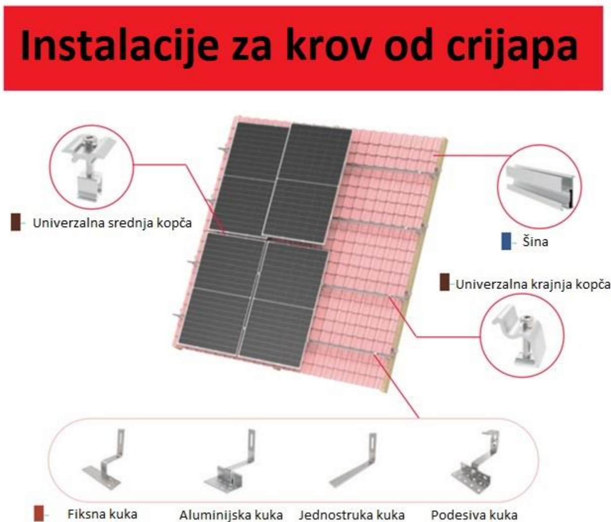
Slika 10.5. Konstrukcija nosača iz kataloga [34]
