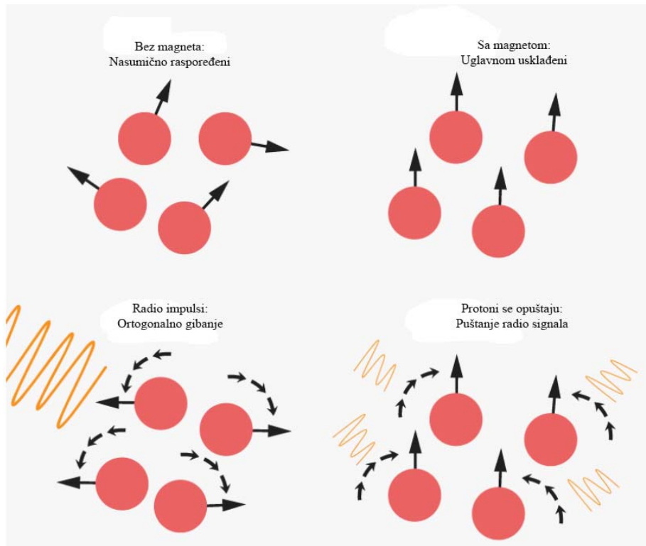
Slika 4.9 Kretanje protona
