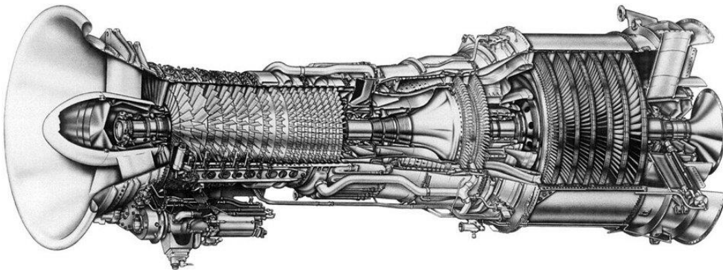
Slika 5.3. Plinska turbina
