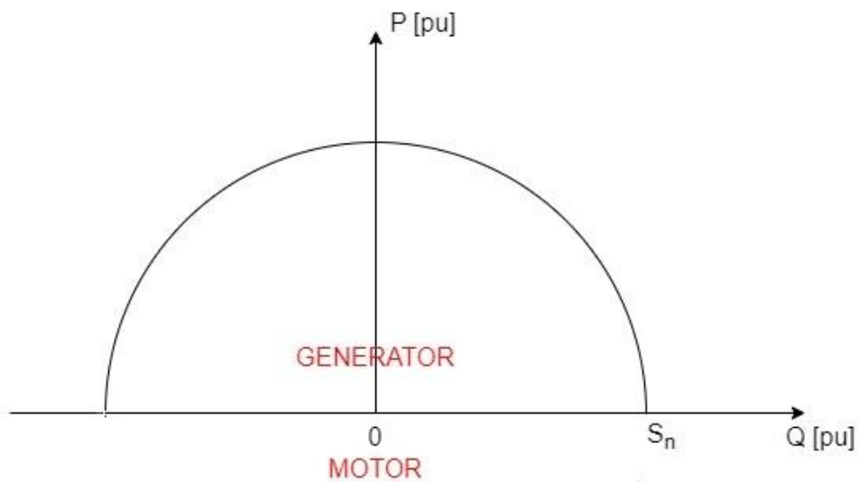
Slika 9.2. Pogonska karta turbogeneratora – jedinična kružnica
