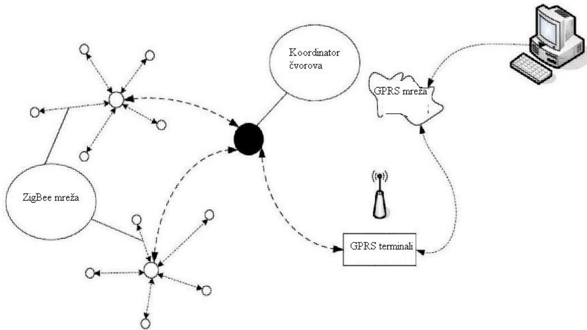
Slika 3.6. Struktura mreže [10]
