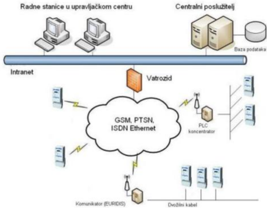
Slika 5.4. AMR sustav [14]
