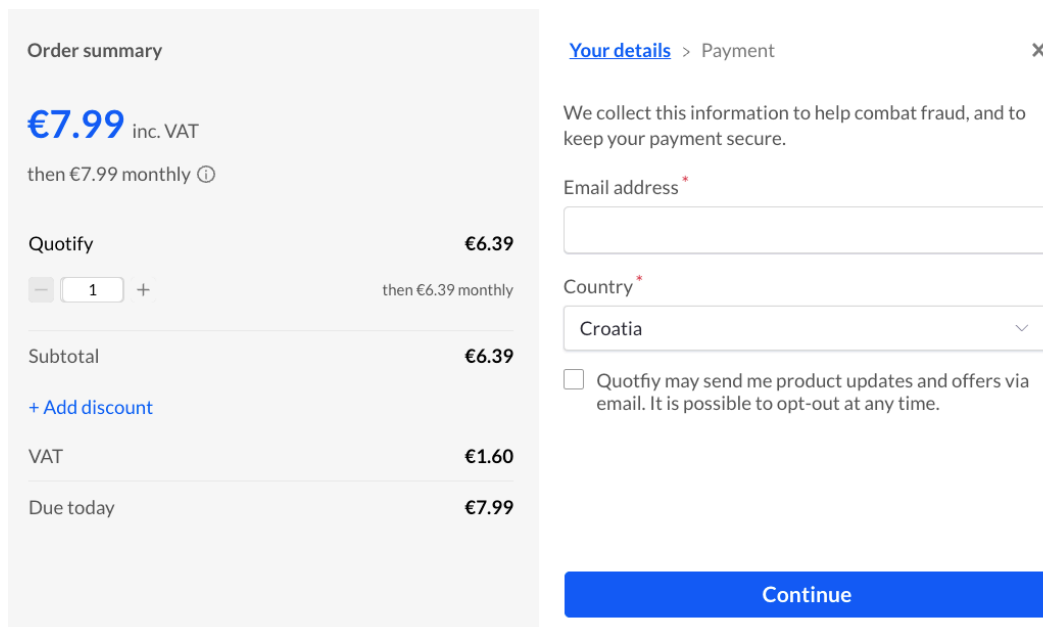
Slika 3.9 – Checkout – korak 1
