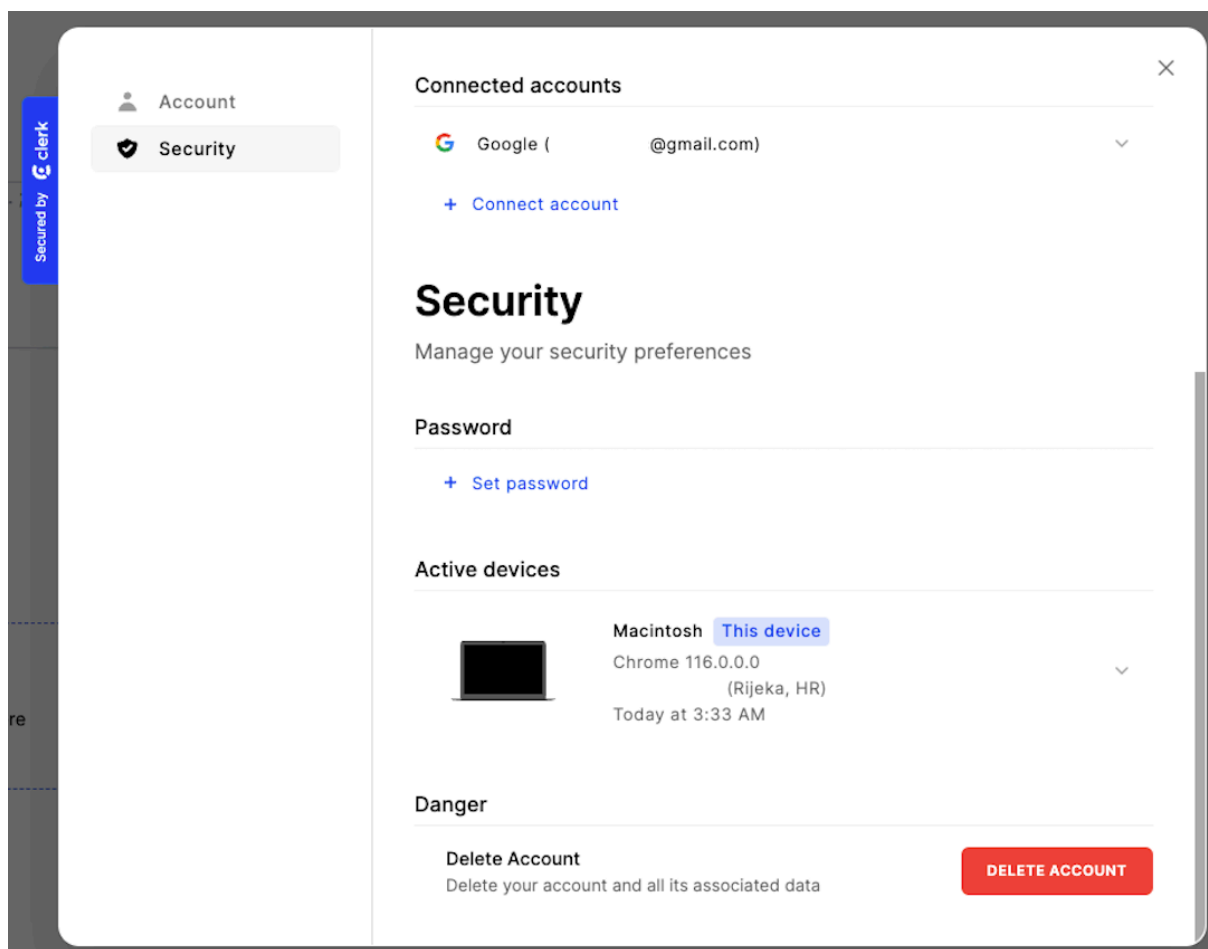
Slika 3.7 – Sigurnosne postavke
