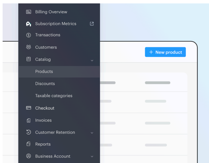
Slika 4.1 – Kreiranje proizvoda
