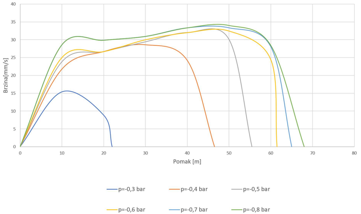
Slika 4.12. Dijagram ovisnosti brzine i pomaku mišića 1 opterećenog silom 30 N
