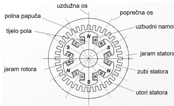
Slika 2.2. Presjek magnetskog kruga s istaknutim 6-polnim uzbuđnim namotom [3]
