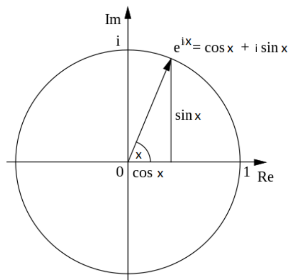
Slika 4.2 Eulerova formula [7]
