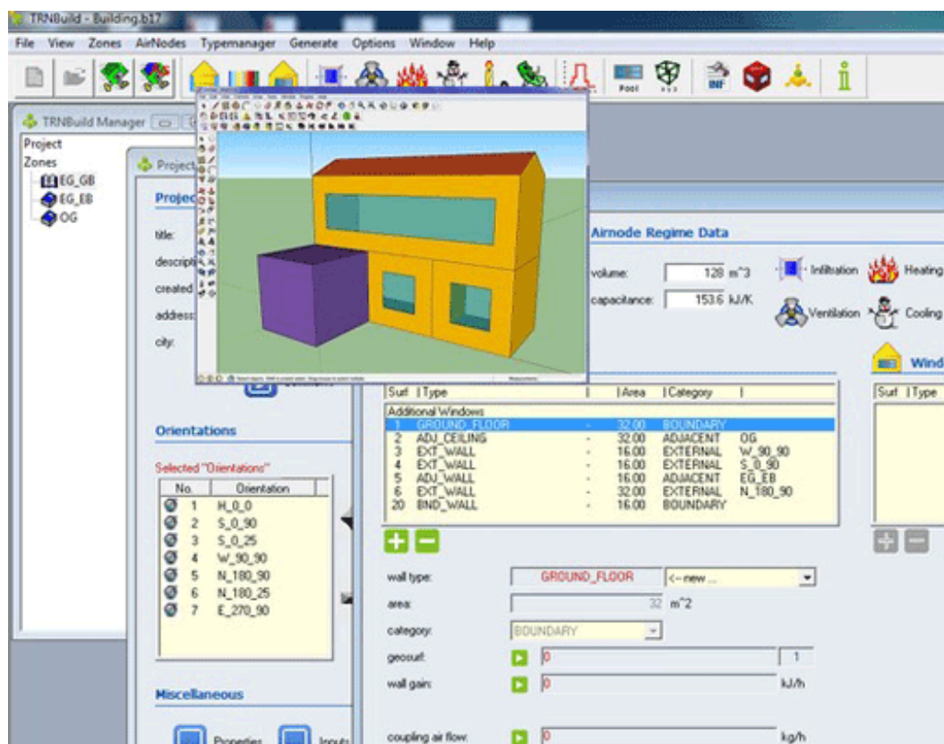
Slika 5.2. TRNBuild alat [12]
