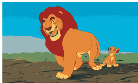
Slika 4.8 k = 10 , RGB
