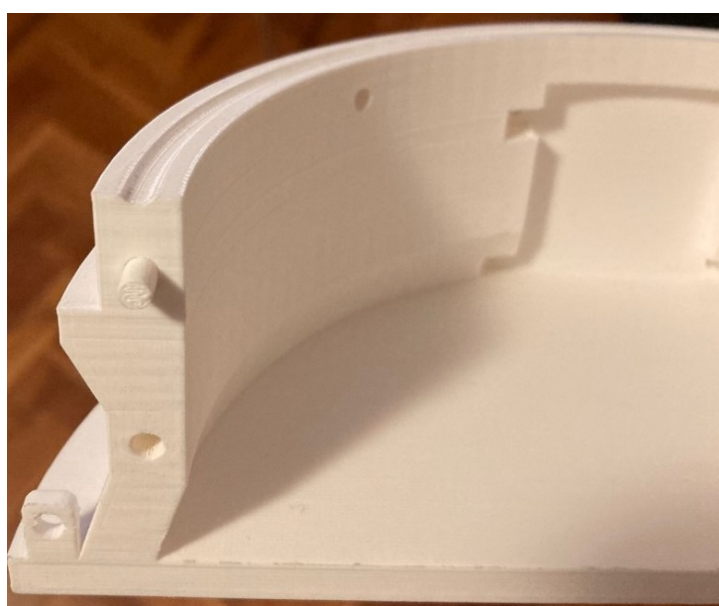
Slika 6.3-Montaža donjeg dijela postolja uz pomoć cilindara
