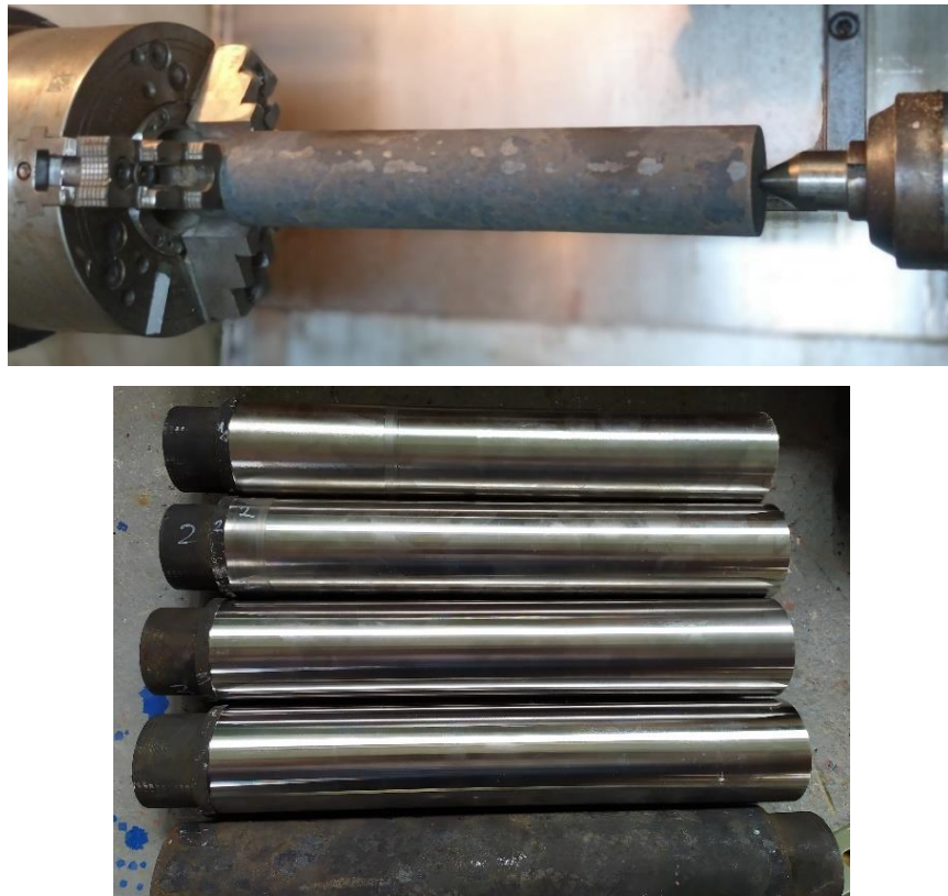
Slika 6.1. Ulazni materijal eksperimenta uz prikaz već obrađenih šipki.
