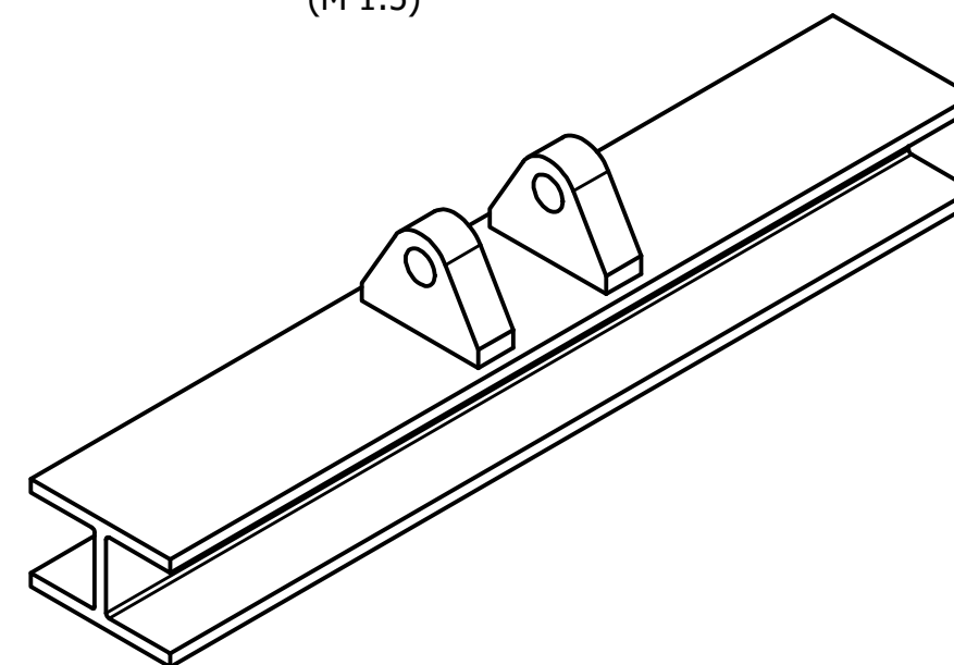
Izometrija (M 1:5)
