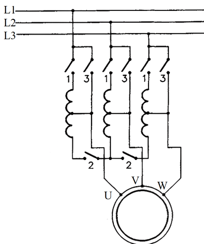
Slika 5.4 Zalet asinkronog motora pomoću autotransformatora [1]
