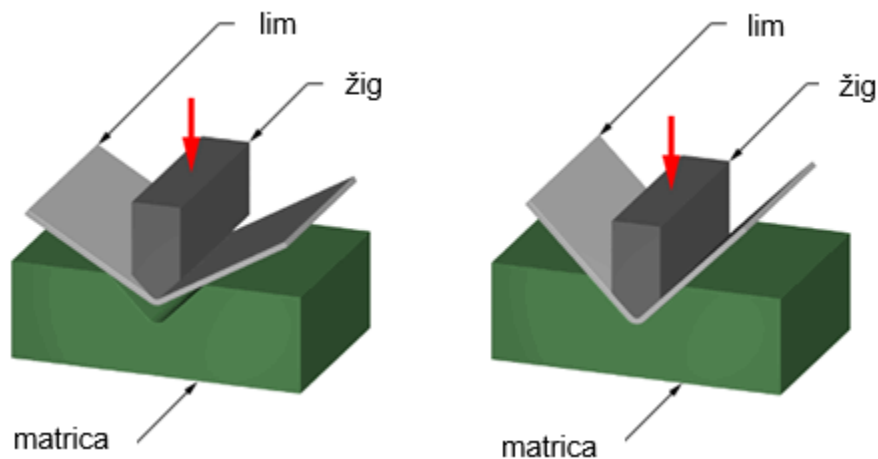
Slika 9. Savijanje V-profila [14]
