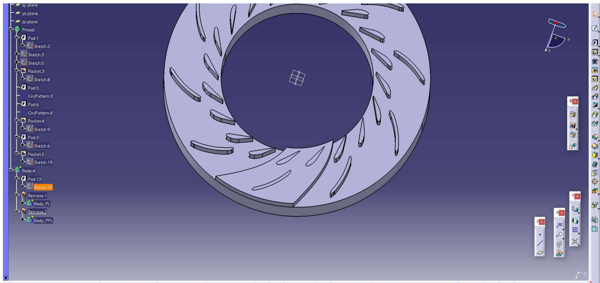
Slika 3.16. Oduzimanje geometrije privoda od geometrije periodičkog kanala
