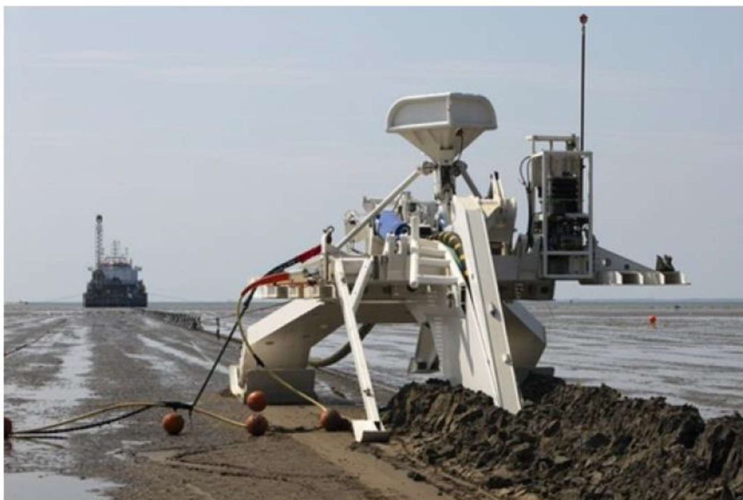
Slika 7.5: Oprema za plug na kopnu [1]
