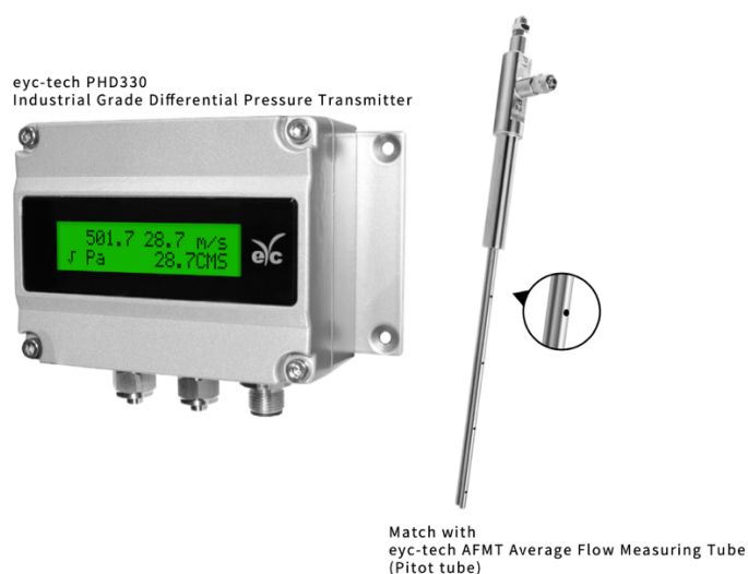
Slika 5.3 Average Pitot cijev i odašiljač „ Differential Pressure – PHD330“ [21]
