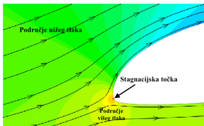
Slika 4.3 Stagnacijska točka [19]
