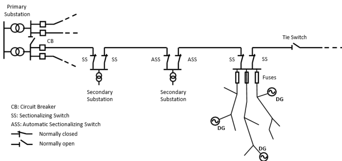
Slika 4.1. Tradicionalna sredjenaponska distribucijska mreža [16]
