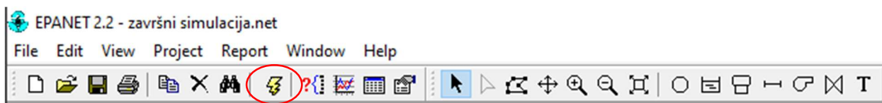
Slika 5.10. Pokretanje simulacije
