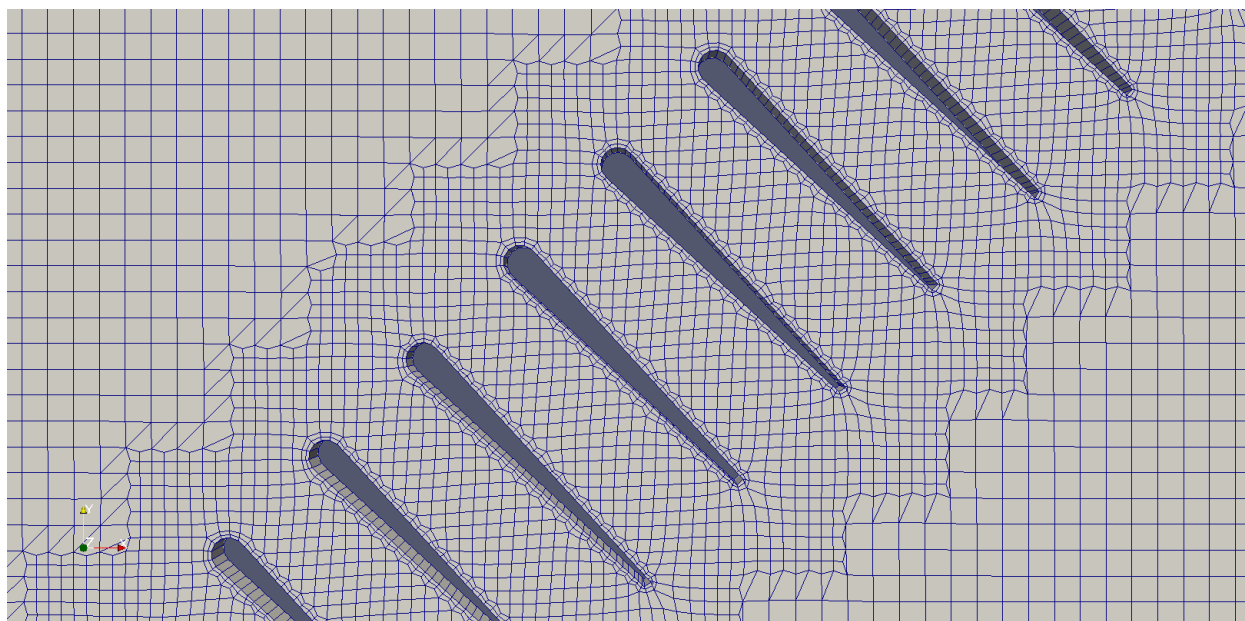
Slika 6.10. Detalj lamela u zaštitnoj rešetki
