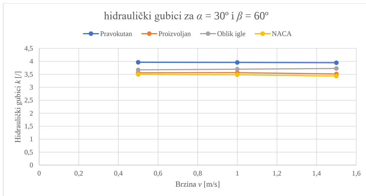
Slika 7.7. Hidraulički gubici u ovisnosti o brzini za \alpha = 30^\circ i \beta = 60^\circ
