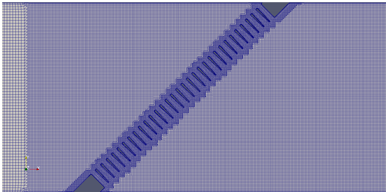
Slika 6.9. Potpuno umrežen model zaštitne rešetke
