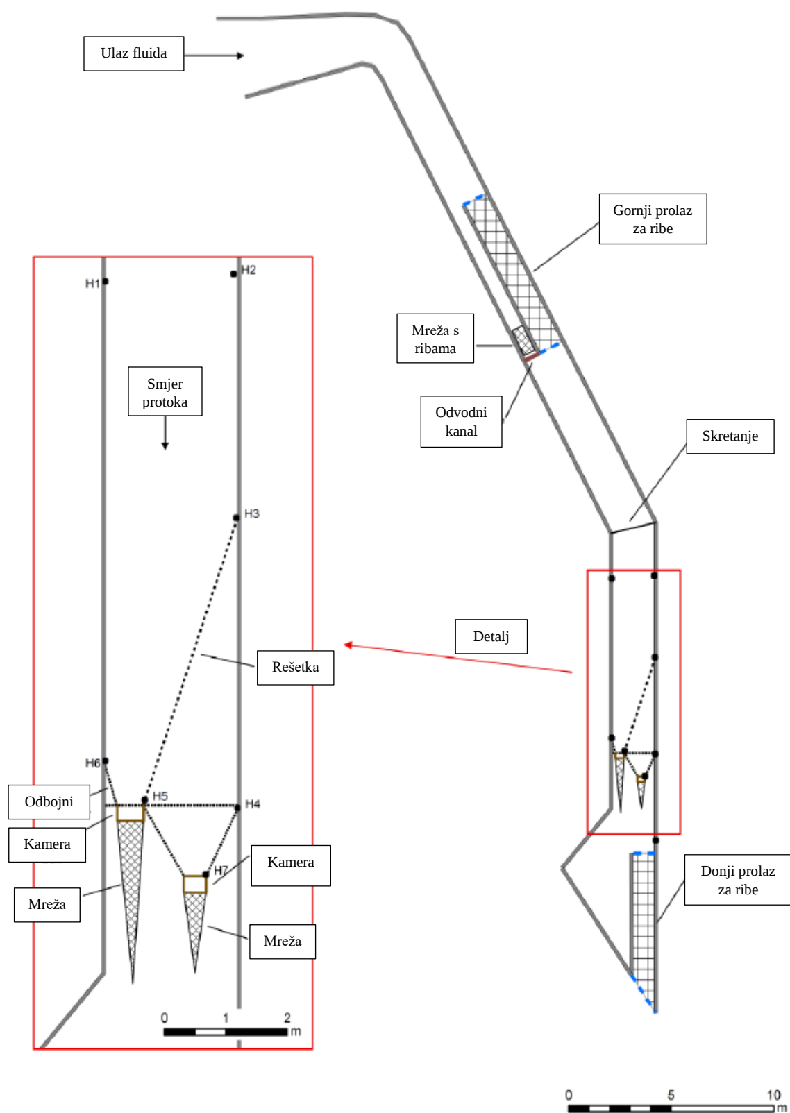
Slika 4.2. Skica eksperimentalnog ispitivanja [9]
