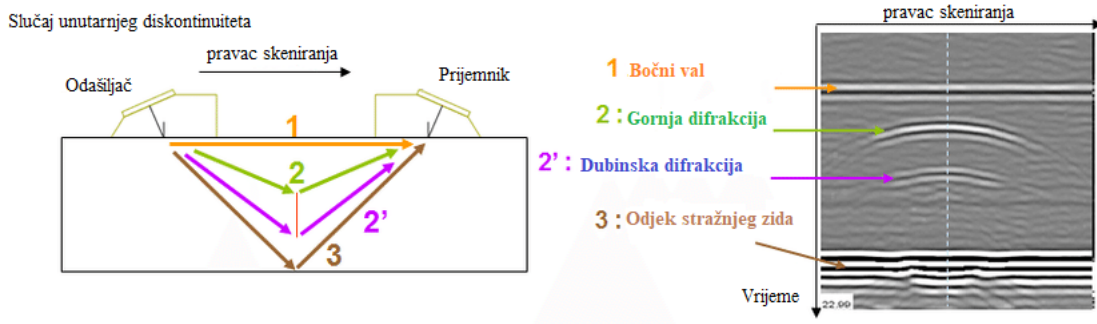
Slika 5.4. Ispitivanje vremena difrakcije leta TOFD pomoću dva ultrazvučna pretvornika
