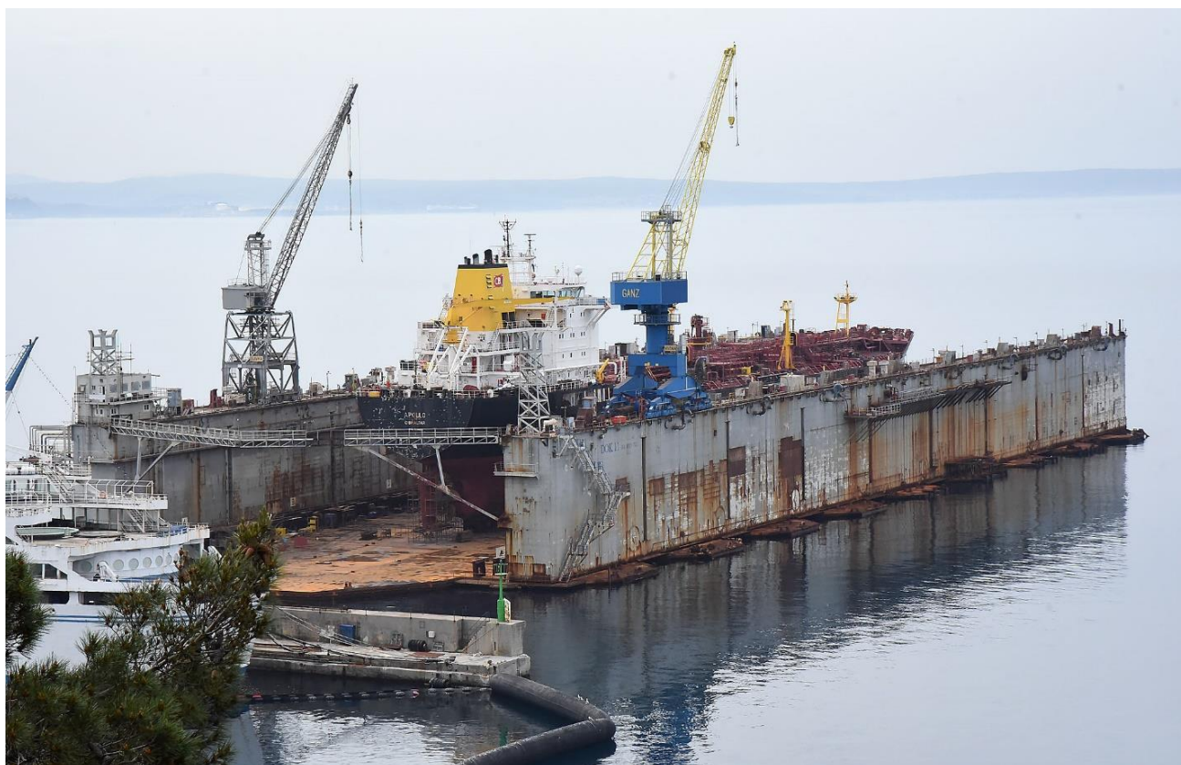
Slika 2.3. Plutajući dok
