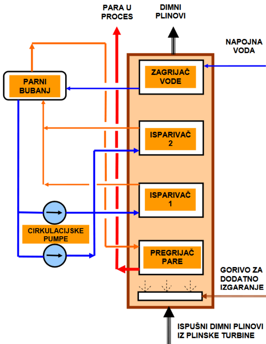
Slika 3.9 Shema utilizatora[14]
