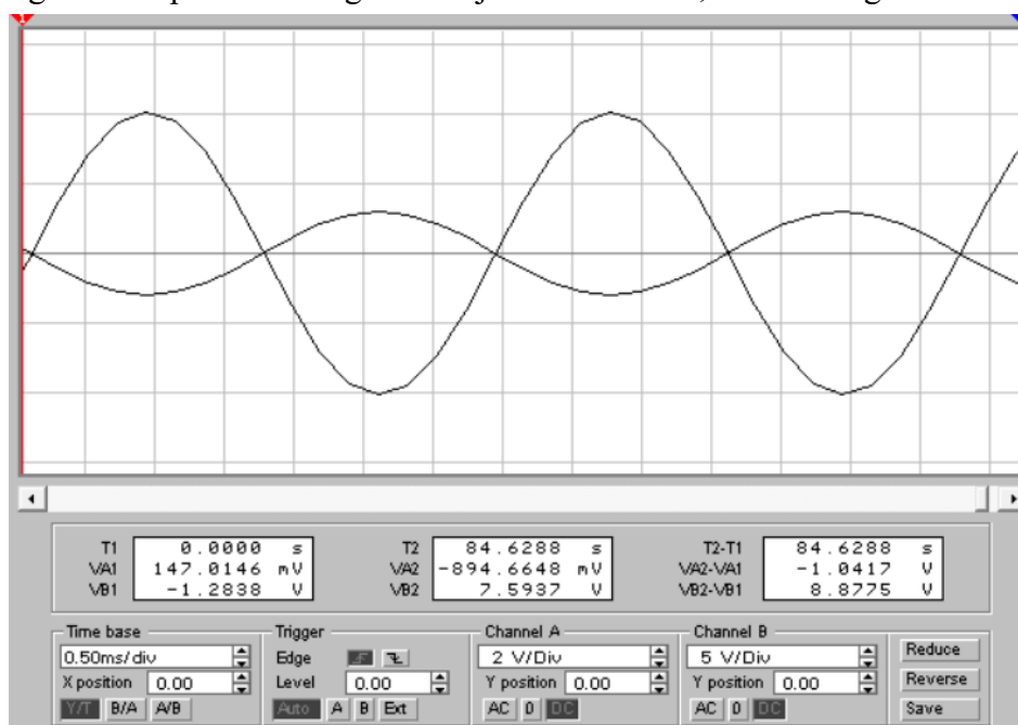
Slika 5.3. Oscilogram usporedbe ulaznog i izlaznog signala sklopa
