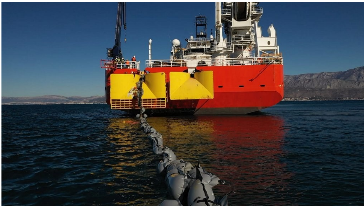
Slika 4.11. Polaganje na obalnom području pomoću plutajućih balona [21]
