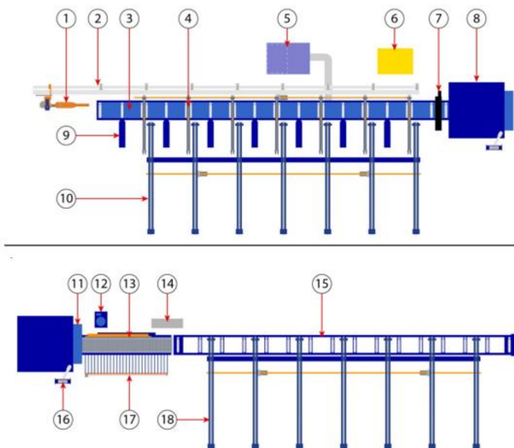
Slika 15.2 Prikaz profil linije
