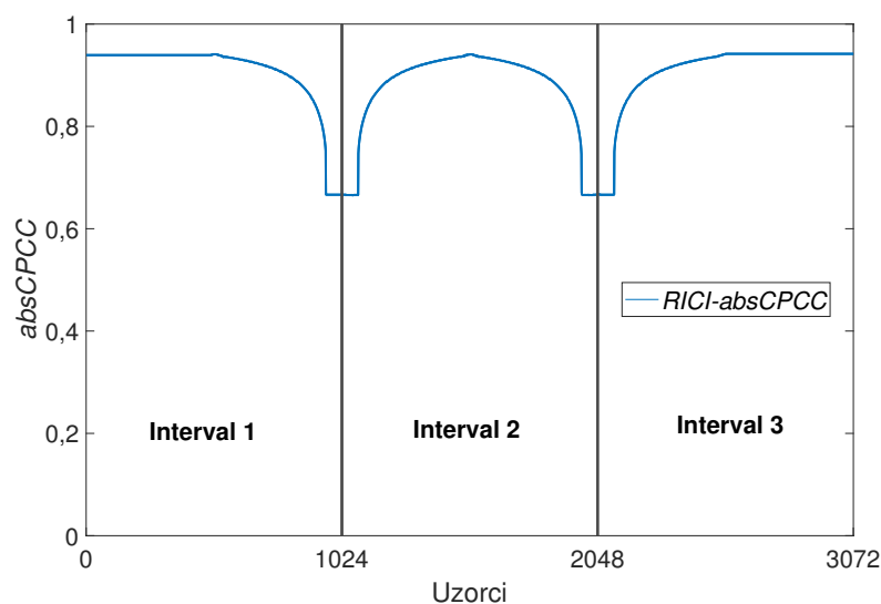
Slika 5.8: Procjena dinamičke funkcionalne povezanosti korištenjem RICI-absCPCC metode.
