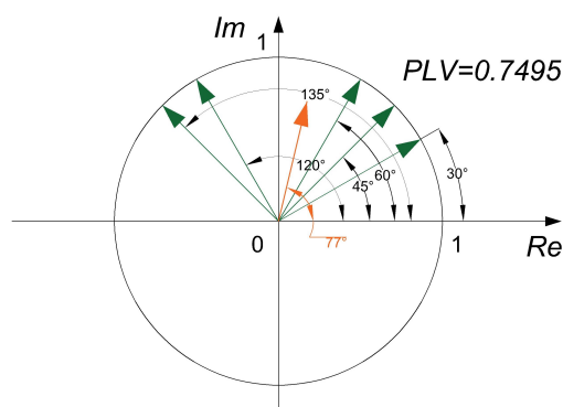
Slika 2.3: Vizualizacija usrednjavanja korištenog pri izračunu PLV -a. PLV se izračunava iz jediničnih vektora koji predstavljaju trenutne fazne razlike.
