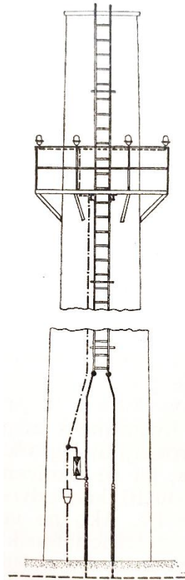
Slika 7.4. Gromobranska instalacija tvorničkog dimnjaka [1]
