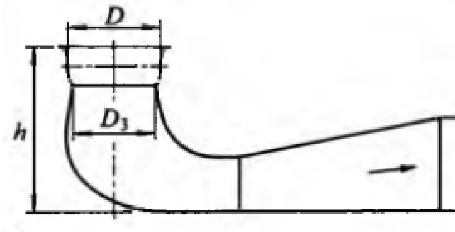
Slika 3.3. Koljenasti difuzor [5]
