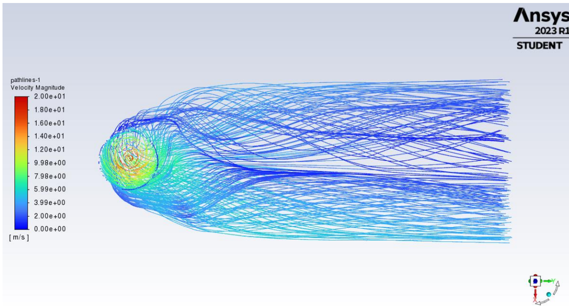
Slika 7.11. Tlocrt kontura strujanja za originalni difuzor
