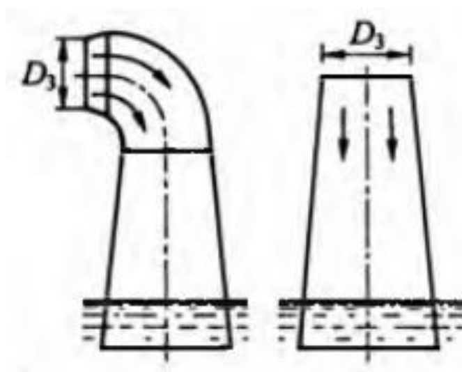
Slika 3.2. Stožasti (lijevo) i ravni (desno) konični difuzor [5]
