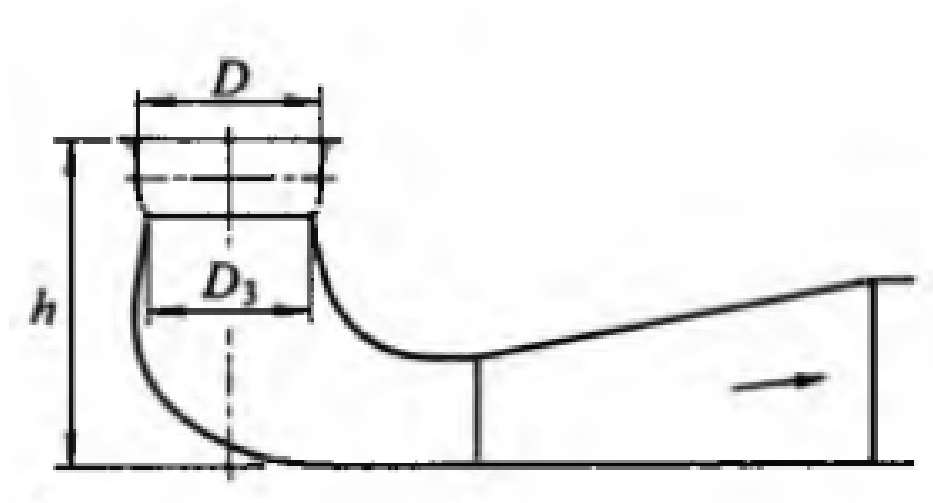
Slika 3.3. Koljenasti difuzor [5]
