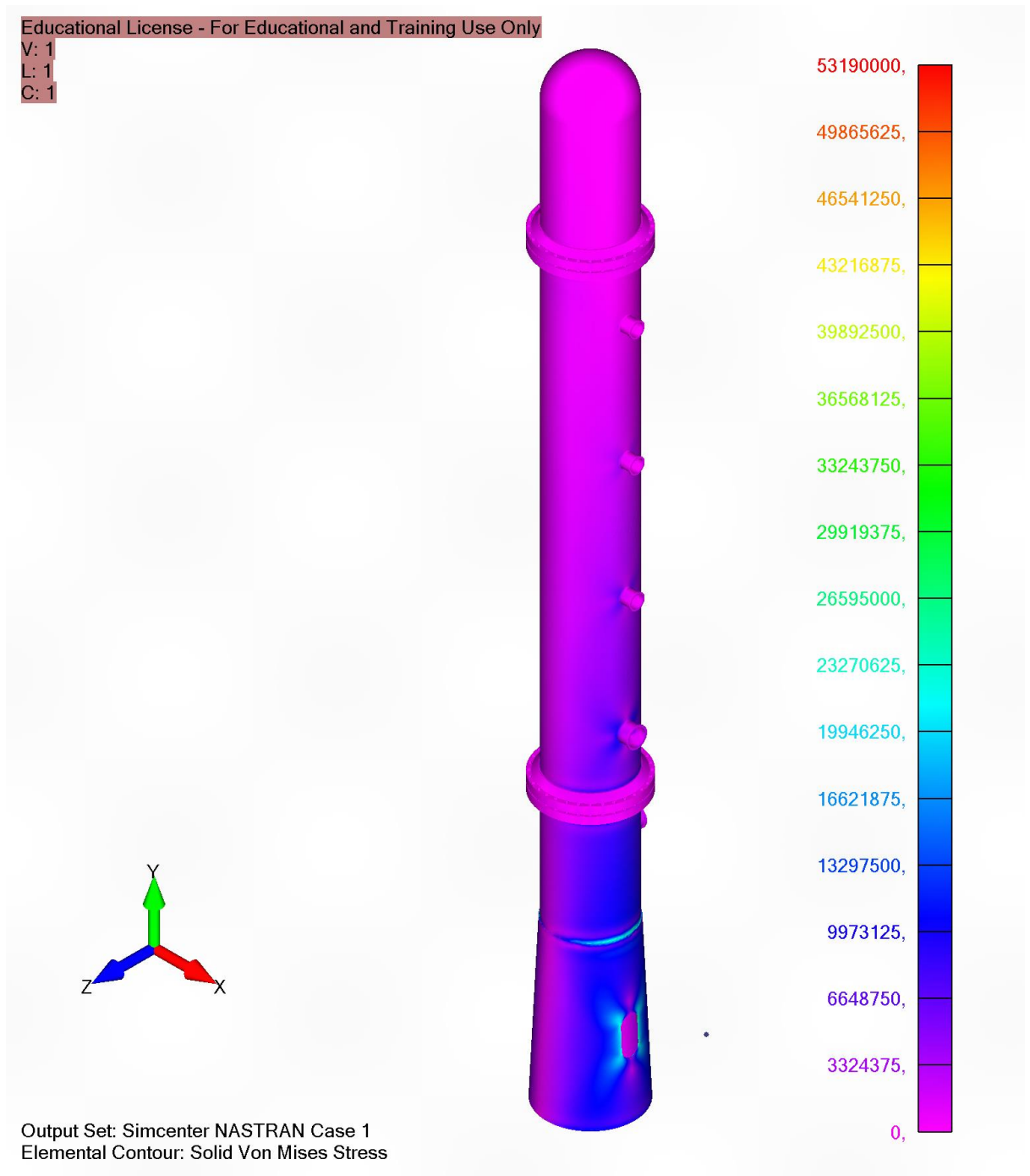
Slika 4.25 Raspodjela Von Misesovih naprezanja na cijeloj koloni
