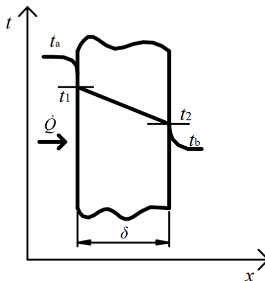
Slika 2.8. Prolaz topline kroz ravnu stijenu
