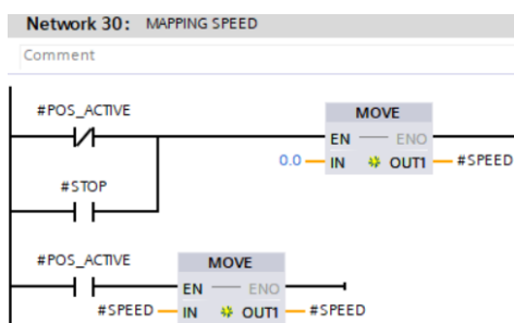
Slika 6.3.24. Mapiranje brzine
