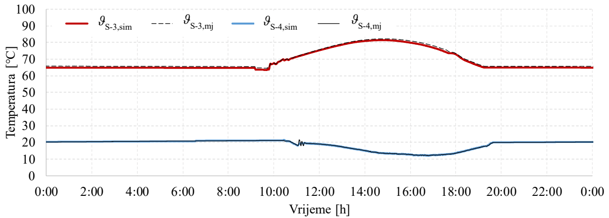
Slika 2.6 Temperatura na vrhu spremnika S-3 i srednja temperatura spremnika S-4
