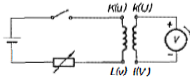
Slika 3.3. Provjera oznaka stezaljki [2]
