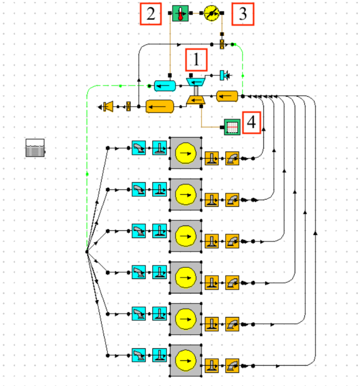
Slika 7.2.1. Shema motora s prednabijanjem
