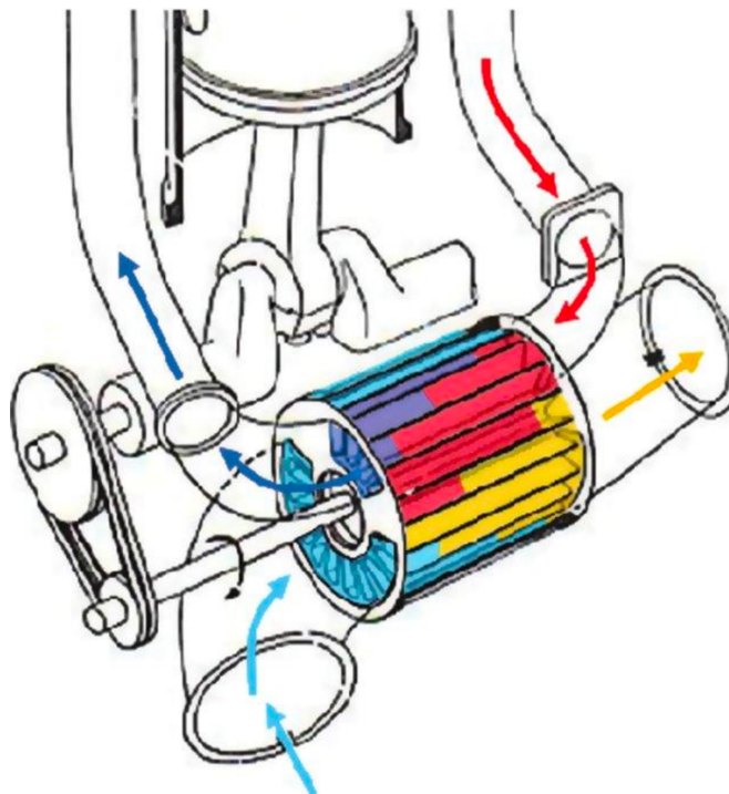
Slika 5.1.2. Vrste prednabijanja [3]
