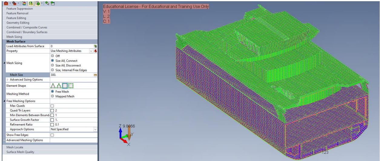
Slika 4.1.1 - Omrežena struktura
