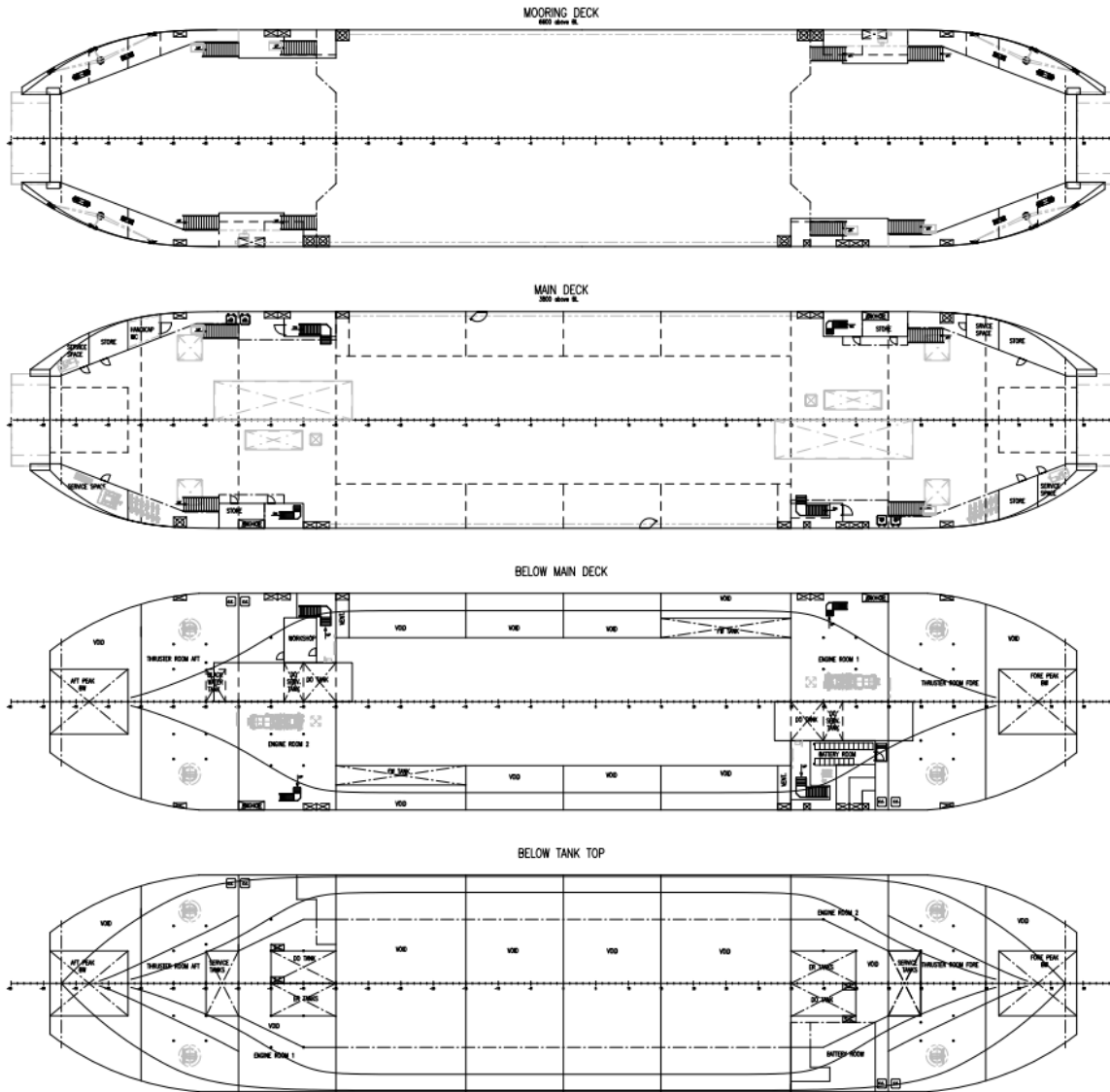
Slika 2.1.2 - Opći plan
